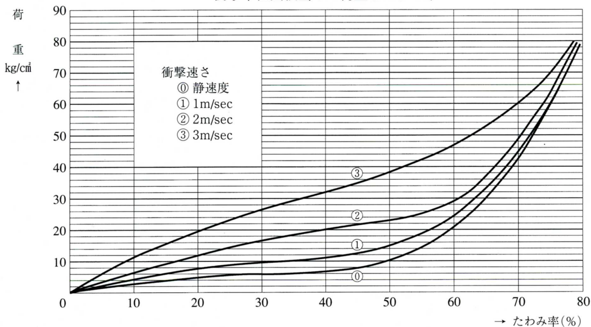
衝撃単位面積当りの荷重とたわみ率
