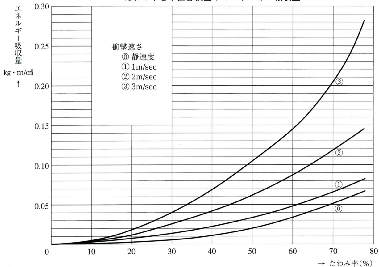
たわみ率と単位容積当りのエネルギー吸収量
